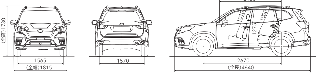
3面図(Advance・ルーフレール装着車) 単位:mm
