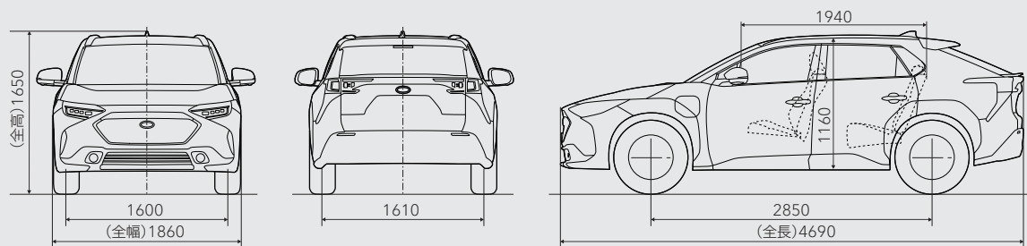
3面図(ET-HS) 単位:mm
